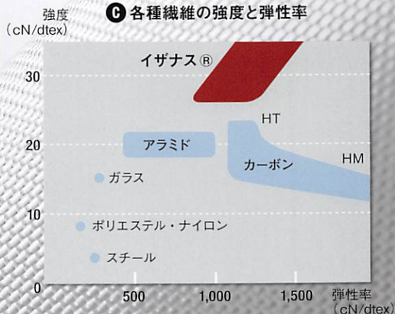
▲C 各種繊維の強度と弾性率
