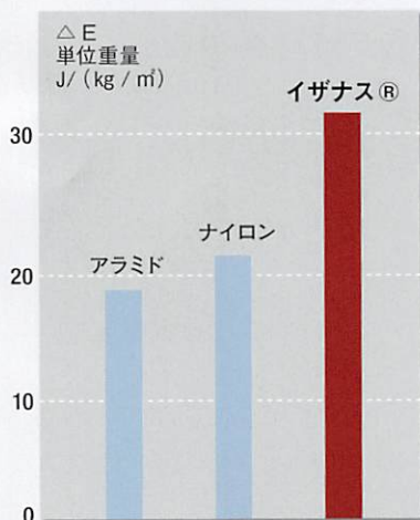
▲A 衝撃エネルギー吸収性
