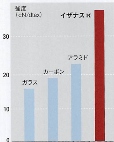
▲B 各種繊維の強度比較
