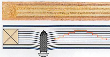
スーパープライコア天板断面図
