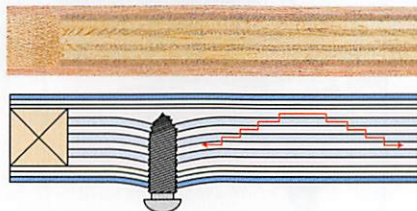
スーパープライコア天板断面図
